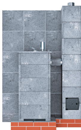
Рис. 9 Пример установки печи с отдельно стоящим дымоходом
