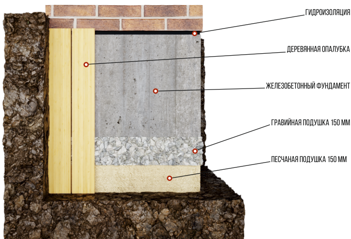
Рис. 13 Схема устройства фундамента
