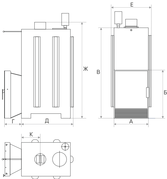
Рис. 1 Габаритные размеры печи
