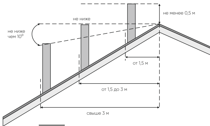
Рис. 14 Возвышение дымохода над кровлей
